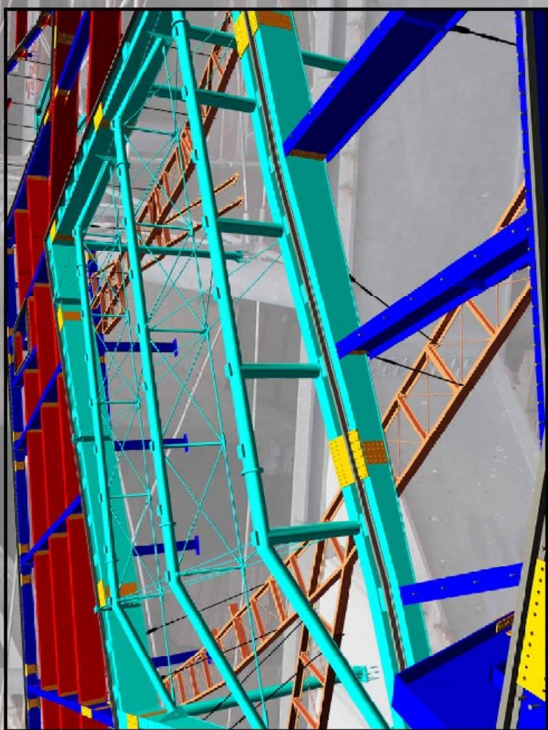
PARTI COLARE CASSONE E ATTACCO DELLA PASSERELLA PEDONALE
